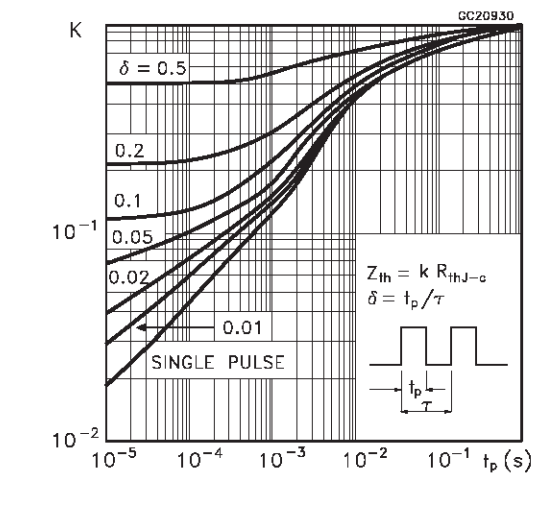
Thermal Impedance
