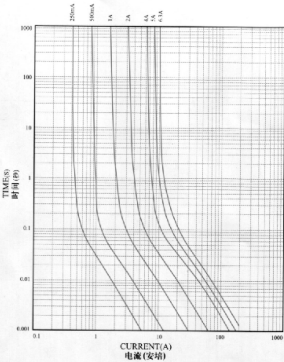
I-T CHARACTERISTICS CURVE 电流-时间曲线图
