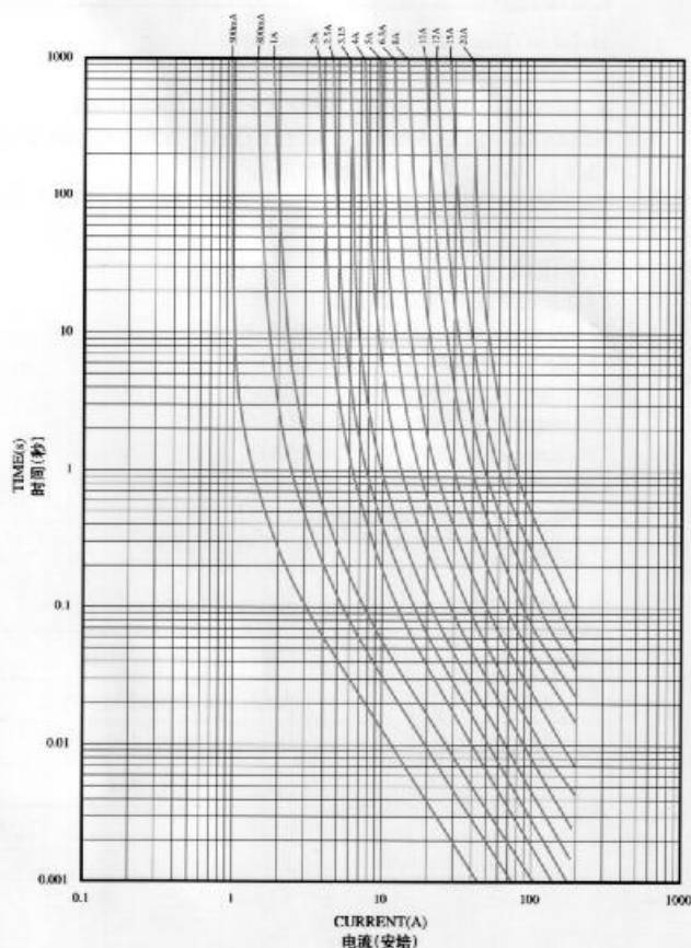
61T RoHS I-T CHARACTERISTICS CURVE 61T RoHS 电流-时间曲线图
