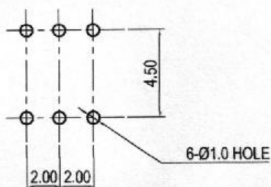
P.C.B LAND PATTERN
