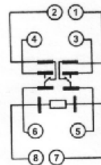
外型圖 開孔尺寸 接線圖 (OUTLINE) (DRILLING PLAN) (WIRING DIAGRAMS)
