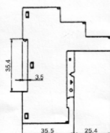
外型圖 開孔尺寸 接線圖 (OUTLINE) (DRILLING PLAN) (WIRING DIAGRAMS)
