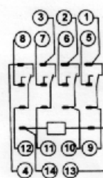
外型圖 開孔尺寸 接線圖 (OUTLINE) (DRILLING PLAN) (WIRING DIAGRAMS)
