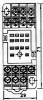
外型圖 開孔尺寸 接線圖 (OUTLINE) (DRILLING PLAN) (WIRING DIAGRAMS)
